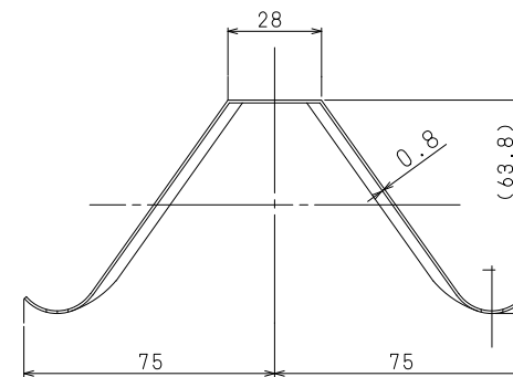
板厚 t0.8
